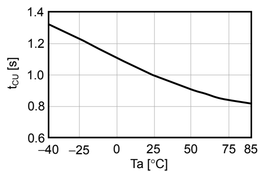
2.12 t_{CU} - Ta
