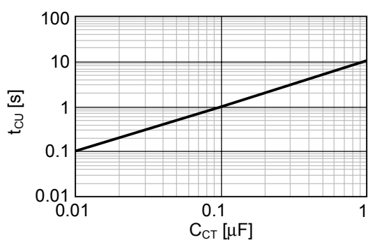
2.11 t_{CU} - C_{CT}
