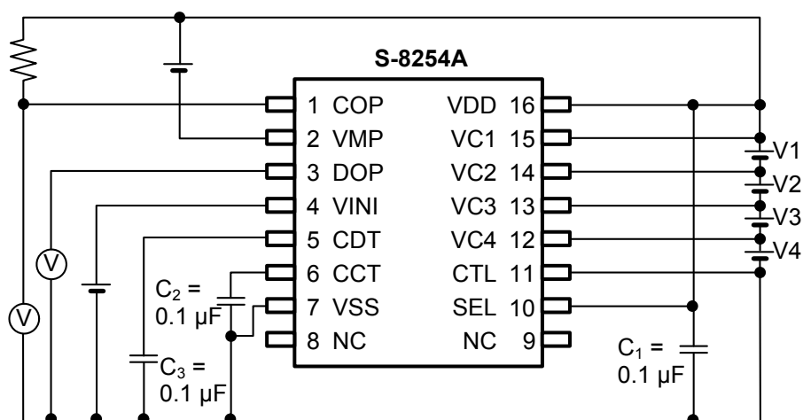
图5 测定电路3
