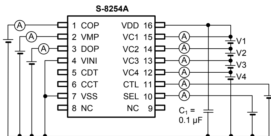
图7 测定电路5
