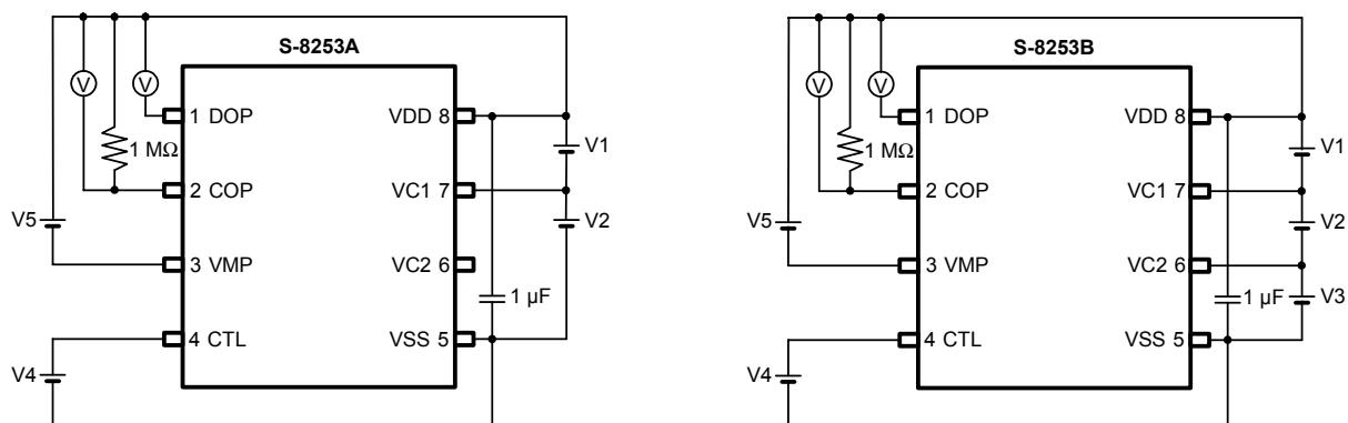
图4 测定电路1
