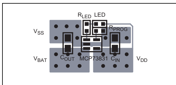
图 6-4: 典型布局 (顶层)
