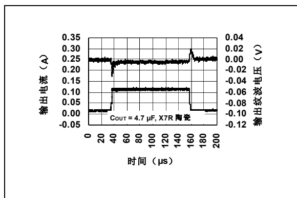
图 2-15: 负载瞬态响应
