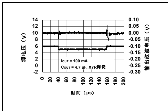
图 2-14: 线性瞬态响应
