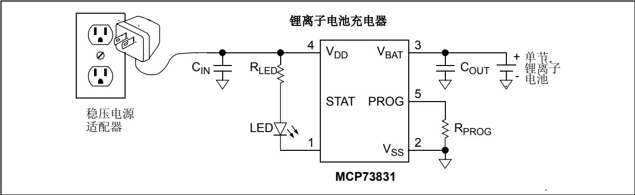
图 6-1: 典型应用电路
