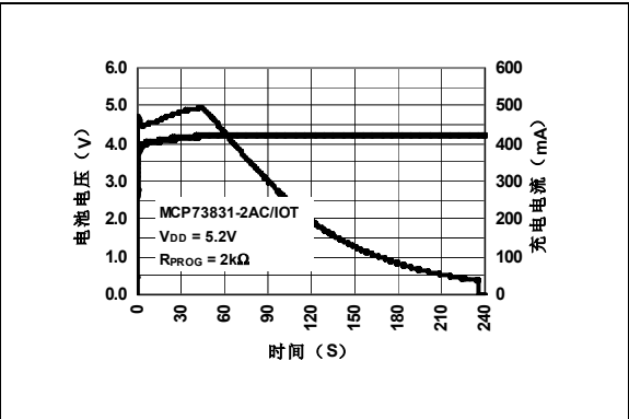
图 6-3: 具有热调节功能的典型充电曲线 (1000 mA 电池)
