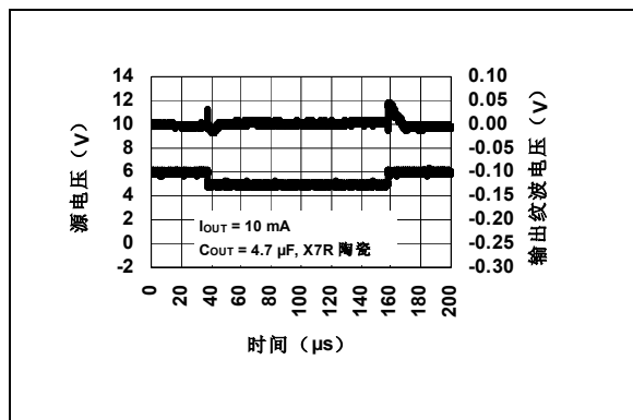
图 2-13: 线性瞬态响应
