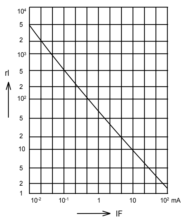
动态正向电阻VS. 正向电流
