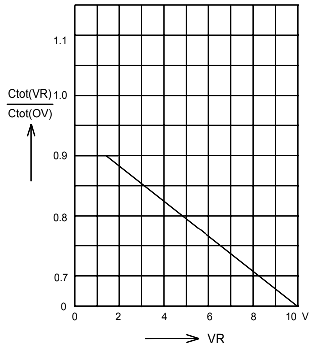
结电容VS. 反向电压
