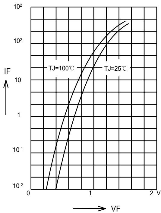
正向特性曲线图
