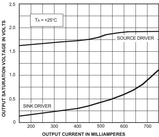
Dwg. GP-064-1A
